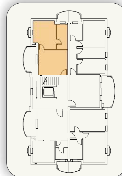
Palazzina A Pianta Piano Secondo Appartamento A6
